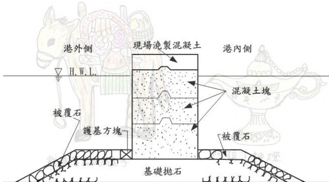
(b) 混凝土塊合成堤
