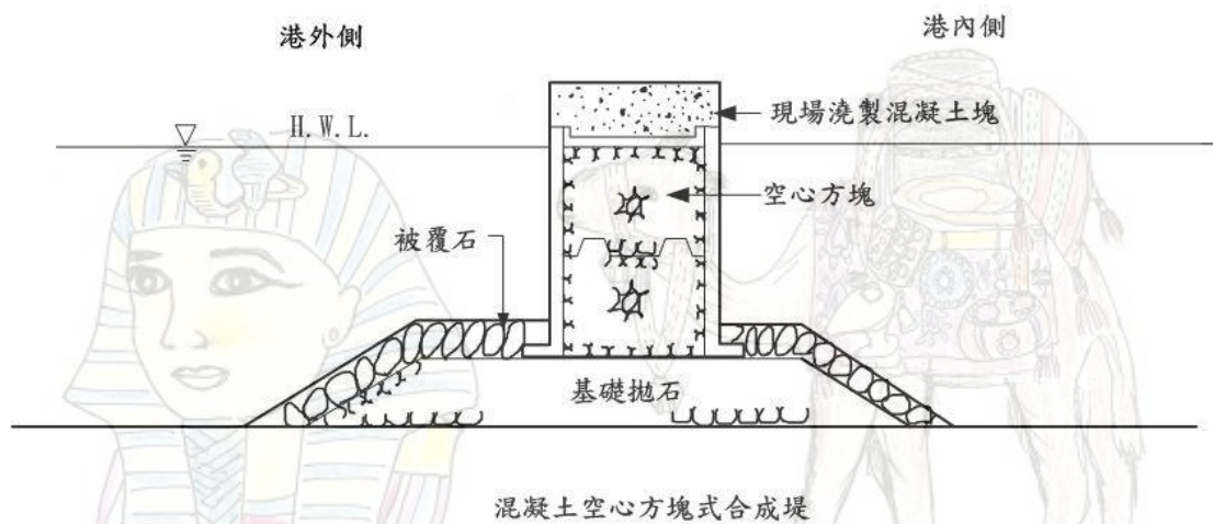
(d) 混凝土塊直立堤
